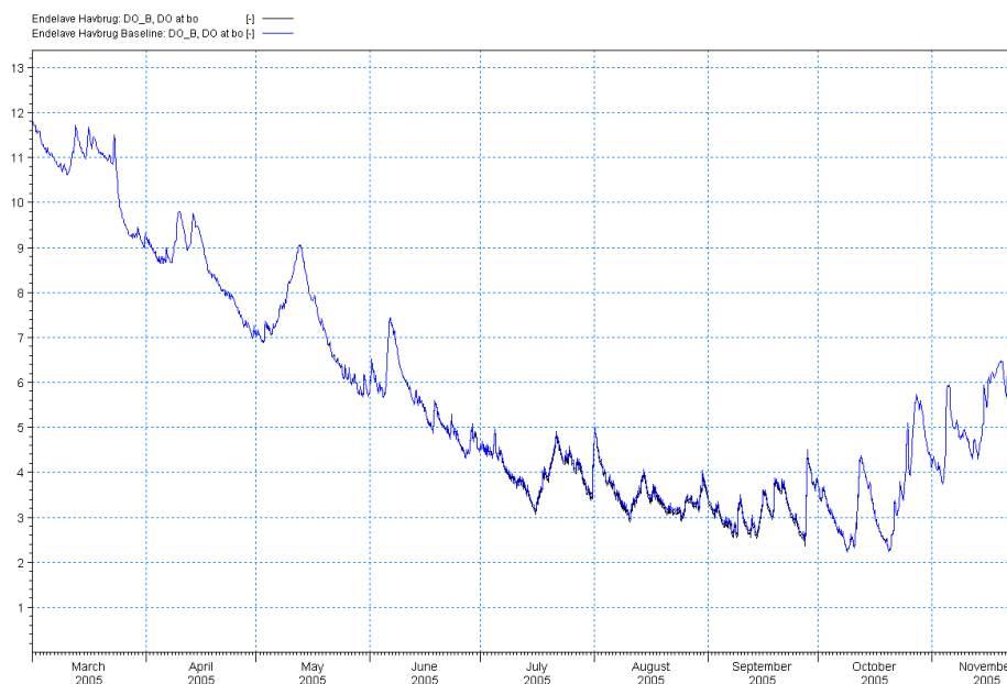
Figur 3.8. Beregnede iltkoncentrationer i bundvandet i projektområdet uden havbrug (basis) og med havbruget etableret. NB: i de tilfælde hvor der kun ses en blå linje betyder det at der er sammenfald i iltkoncentrationerne mellem de to situationer.
