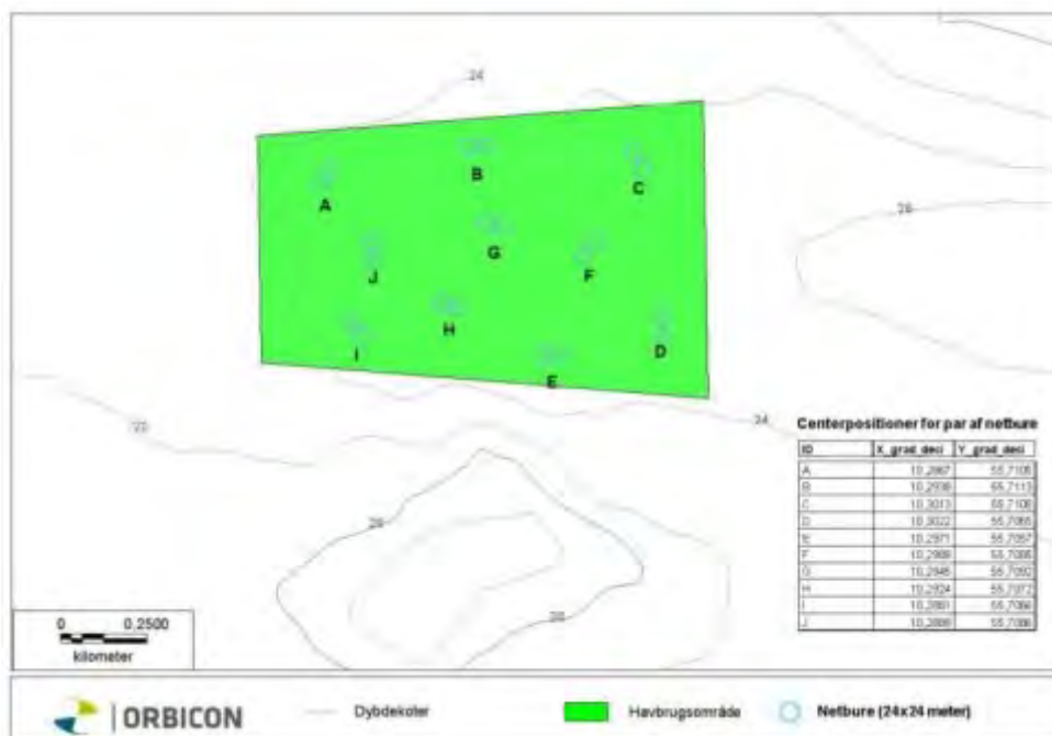
Figur 3.2. Skitse over placeringer af netbure inde i det udlagte projektområde ved Endelave. Området dækker 0,7 x 1,3 km (98 ha).
