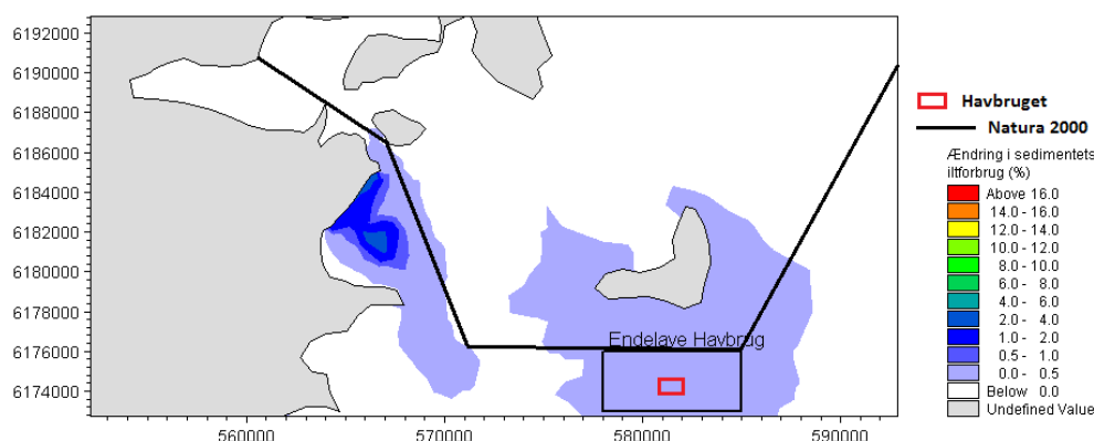
Figur 3.6. beregnet procentvis ændring af sedimentets iltforbrug over en produktionssæson ved etablering af havbrug syd for Endelave og 3 muslingeopdræt i As Vig.
