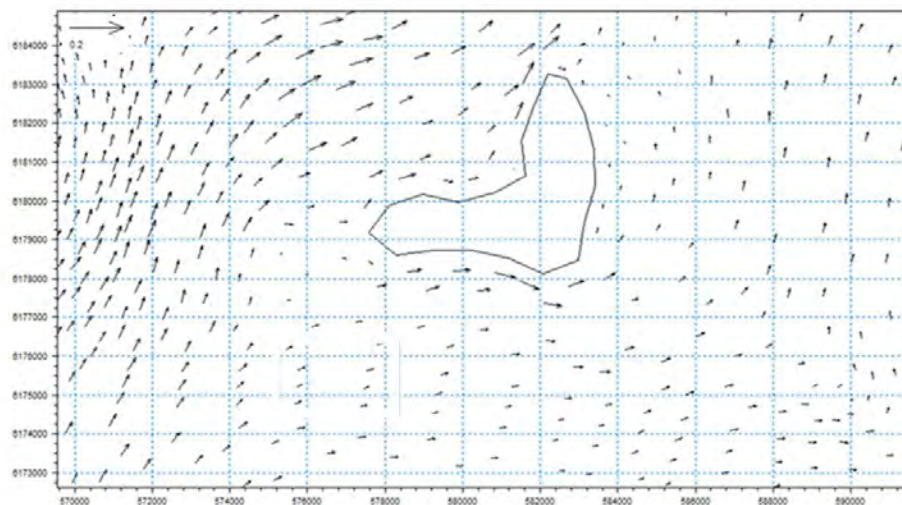
Figur 3.7. Residualstrøm (retning og hastighed) omkring Endelave i perioden 1. april – 30. november 2005. Længden af pil øverst tv. angiver en hastighed på 0,2 m/s. (Møhlenberg, 2011).
